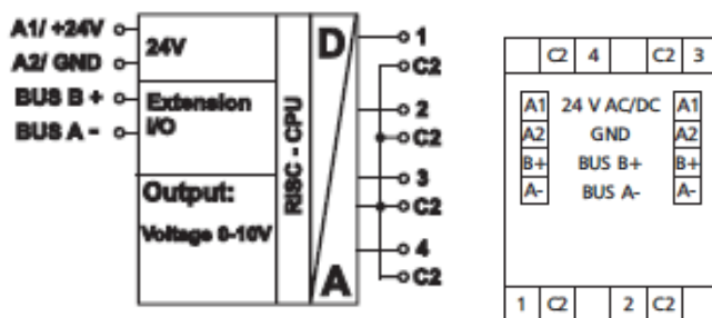
Рис. 1. Монтажная схема и схема подключений
