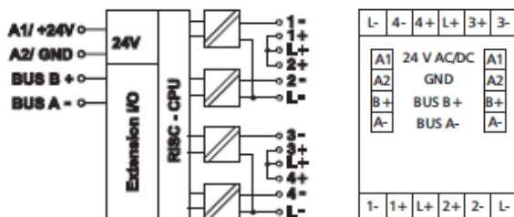
Рис. 1. Монтажная схема и схема подключений
