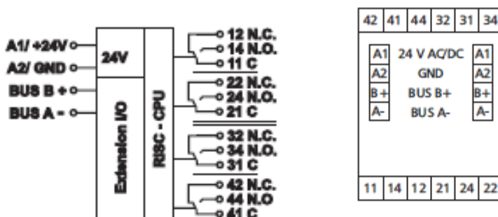
Рис. 1. Монтажная схема и схема подключений
